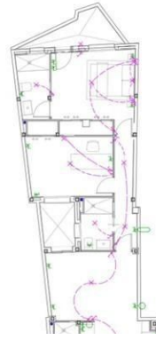
Planta tipo
