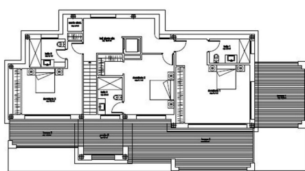
planta alta
