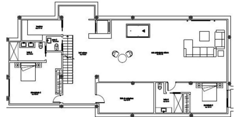
planta sótano
