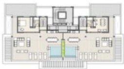
Planta sexta E:1/400
