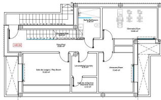
BASEMENT FLOOR (OPCIONAL)
