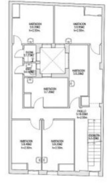
PLANTA PRIMERA SUPERFICIE ÚTIL: 22,81 M 2 SUPERFICIE CONSTRUIDA: 28,36 M 2
