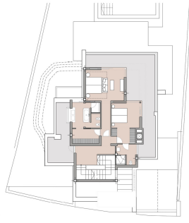
Planta Primera
