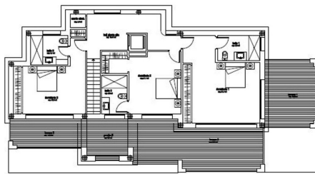
planta alta
