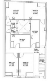
PLANTA PRIMERA SUPERFICIE DEL TERRENO 22,82 M 2 SUPERFICIE CONSTRUIDA 88,36 M 2
