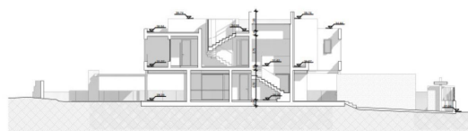
SECCIÓN A-A'
