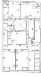
PLANTA PRIMERA
