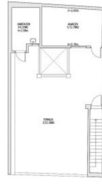
PLANTA CUBIERTA SUPERFICIE ÚTIL: 18,95 M 2 SUPERFICIE CONSTRUIDA: 22,73 M 2
