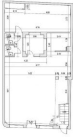
PLANTA BAJA
